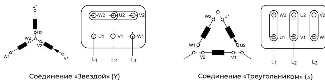
Рис. 6 Примеры трёхфазного подключения электродвигателя
