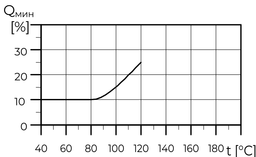
Рис. 10 Пример минимальной подачи насоса BM(N)
