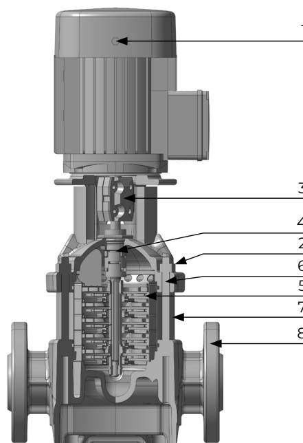
Рис. 1 Конструкция насоса ВМ(Н)(Е):
