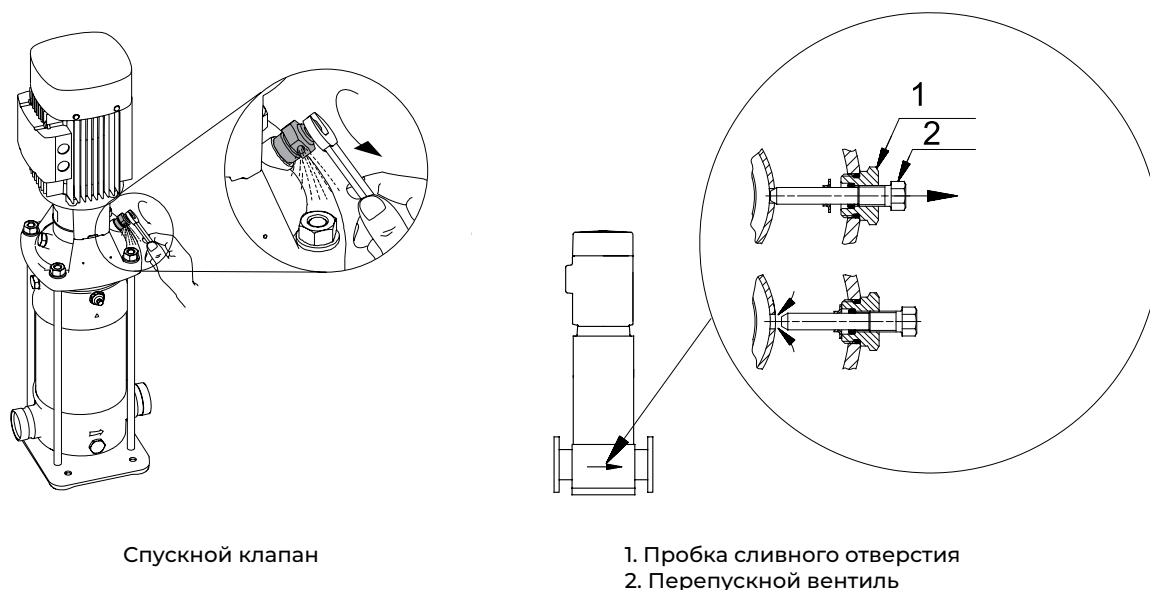
Рис. 8 Спускной клапан воздуха. Перепускной вентиль. Пробка сливного отверстия
