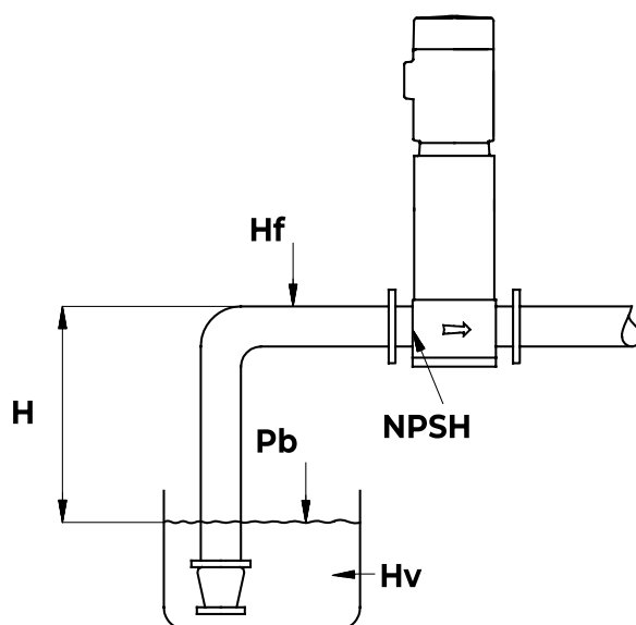
Рис. 9 Пример открытой системы с насосом BM(N)
